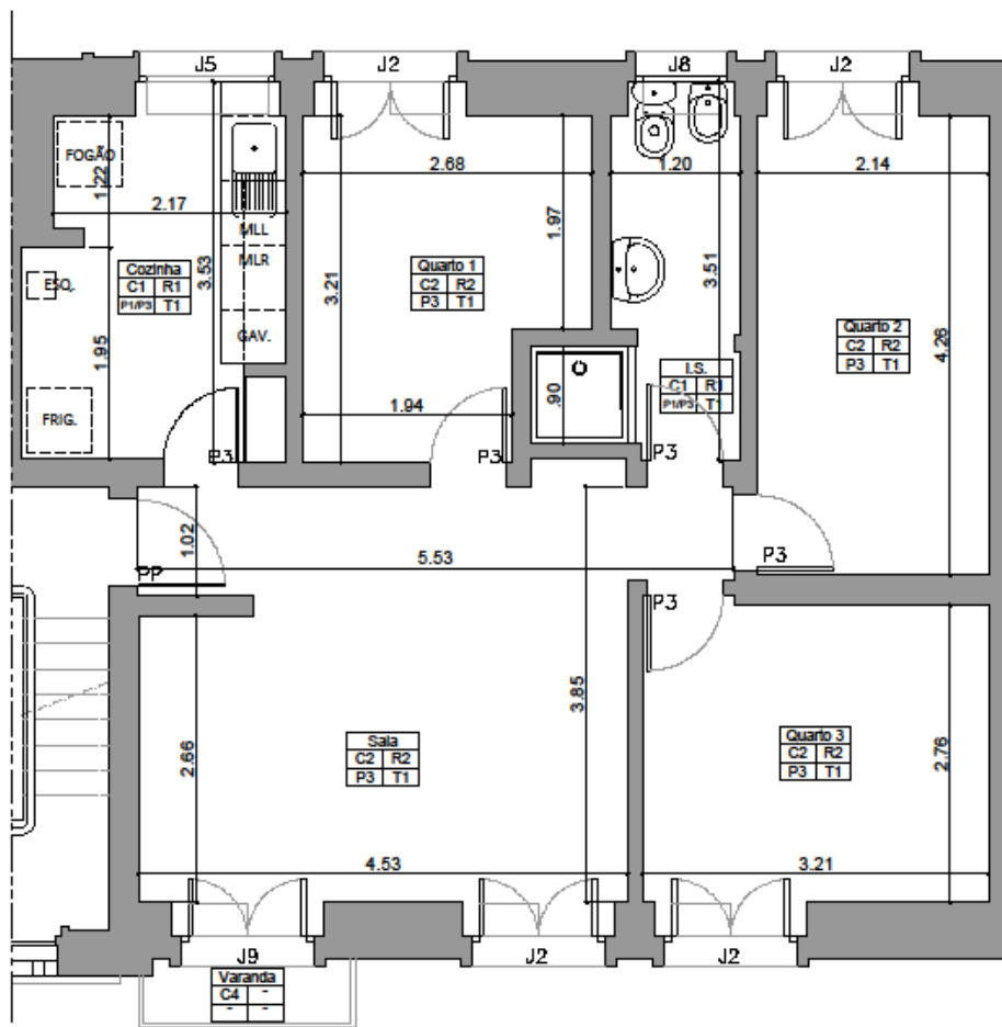
PLANTA
