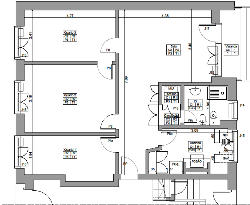
PLANTA
